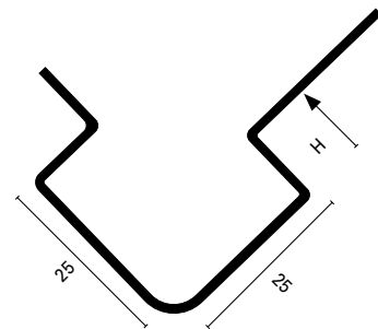
Sezione quotata scala 1:1
